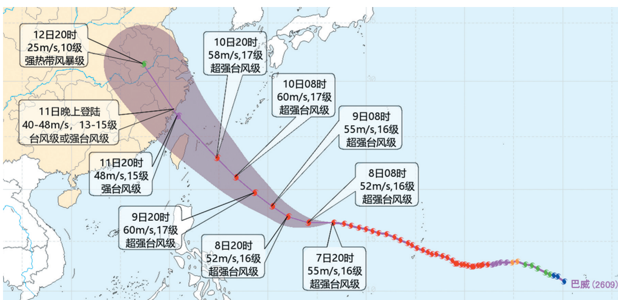
第9号台风“巴威”未来120小时路径概率预报图(中央气象台7月7日21时制作)
