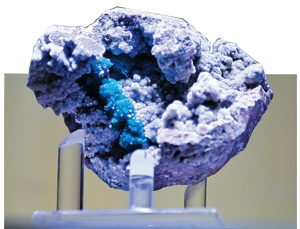
▲水硅矾钙石
