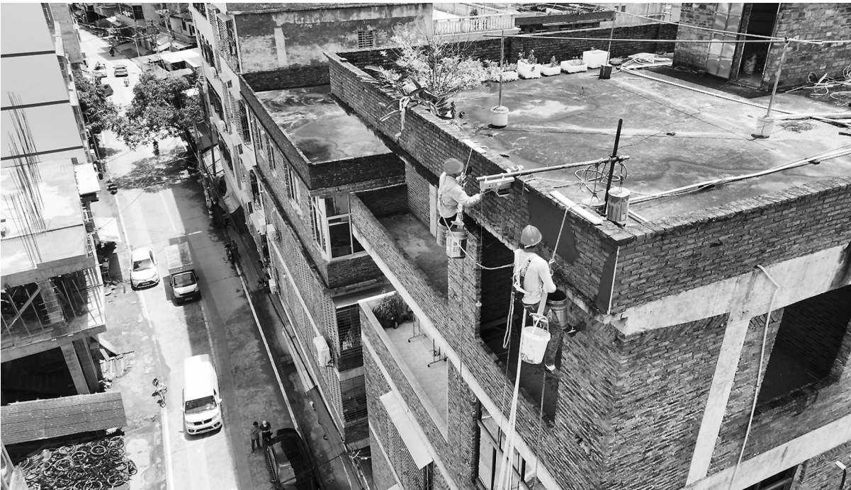
工人正在进行平抹砂浆作业。
