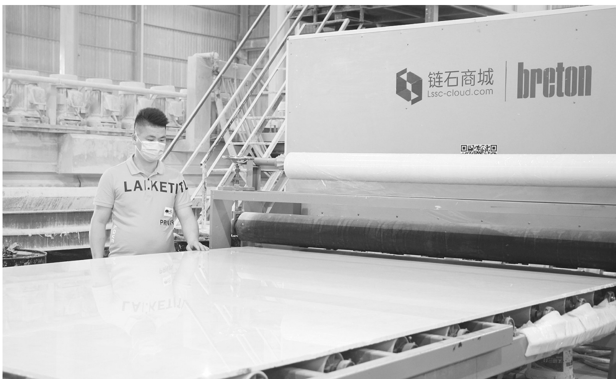
大板经过扫描仪扫描,生成数字大板。
