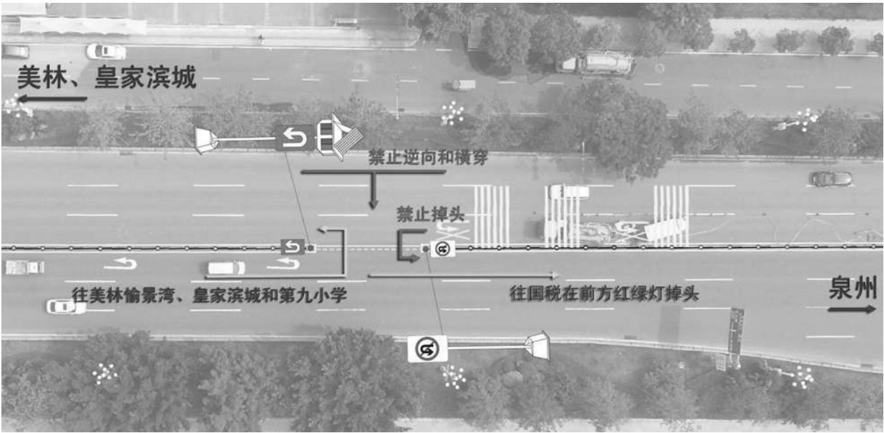
江北大道皇家滨城路段掉头区交通优化示意图。
